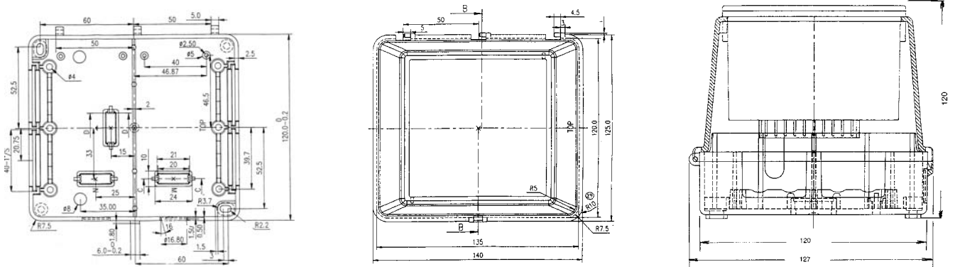
Reglercentral RVA36.531
