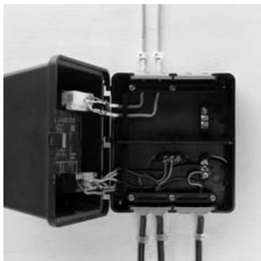
Fig. 3 Montera reglercentralen med bottenplattan. Ledningar drages genom kabelgenomföringar och fästes med dragavlastare mot bottenplattan. Placera ledningarna under kabelhållarna för respektive ledningsgrupp.
